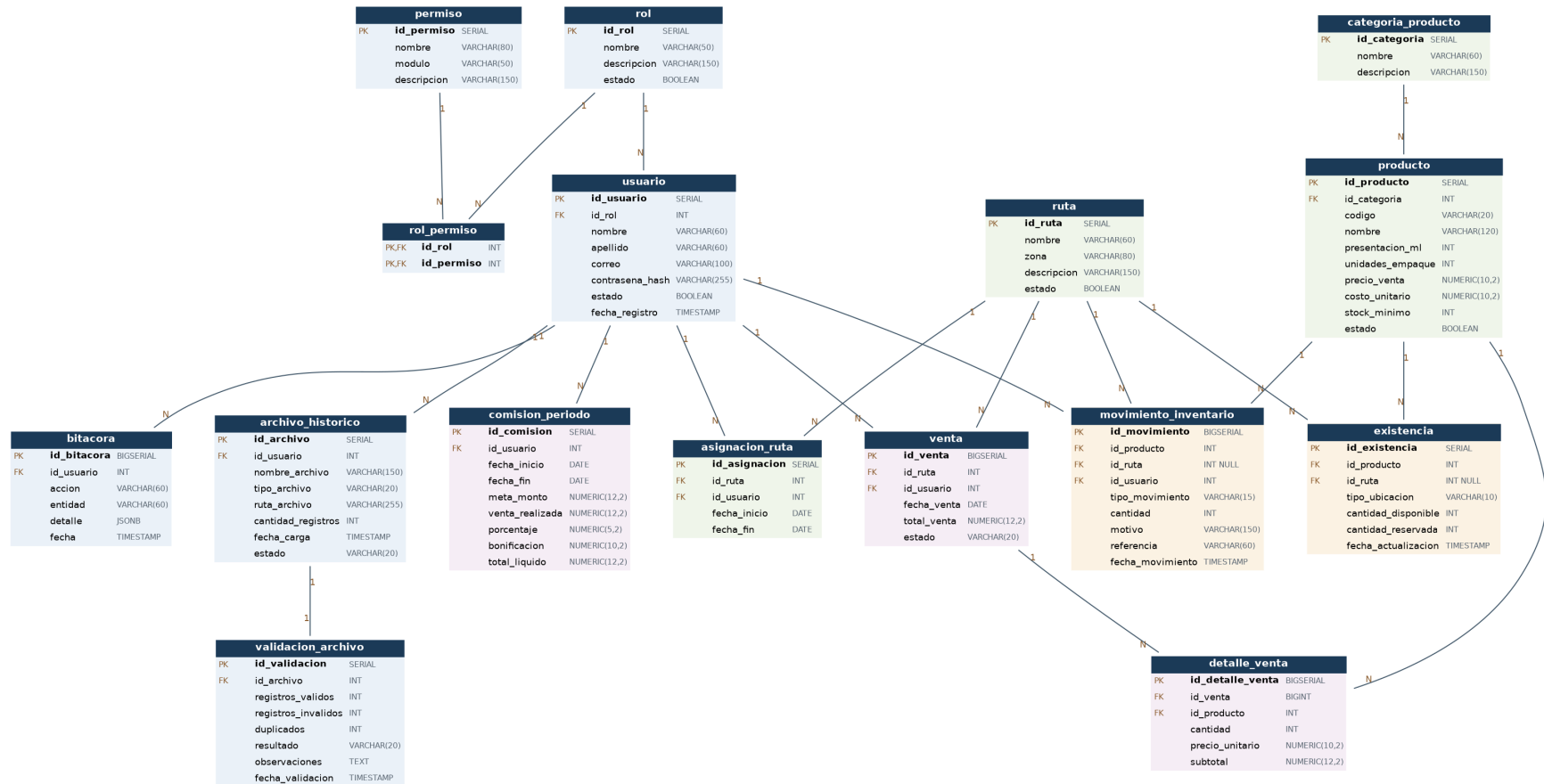
Figura 2. Modelo entidad-relación. Vista 1: seguridad, datos históricos, catálogos, inventario y ventas.
